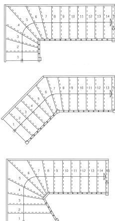
Lukket bøgetrappelpe med vanger i fyr. Klodstrin med rundet forkant.
