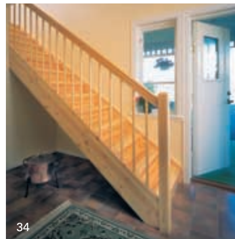
Lige trappe af massiv fyr med stødtrin. Lakeret. Balustre nr. 4, stolpe D1.
