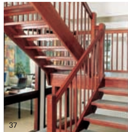
Tilslutning af trappen mod reposen. Vangerne er integreret med siderne af reposen.
