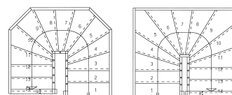
Åbent klodstrin der er rundet i den ene side. I den modsatte side er vangen placeret op mod væggen.
